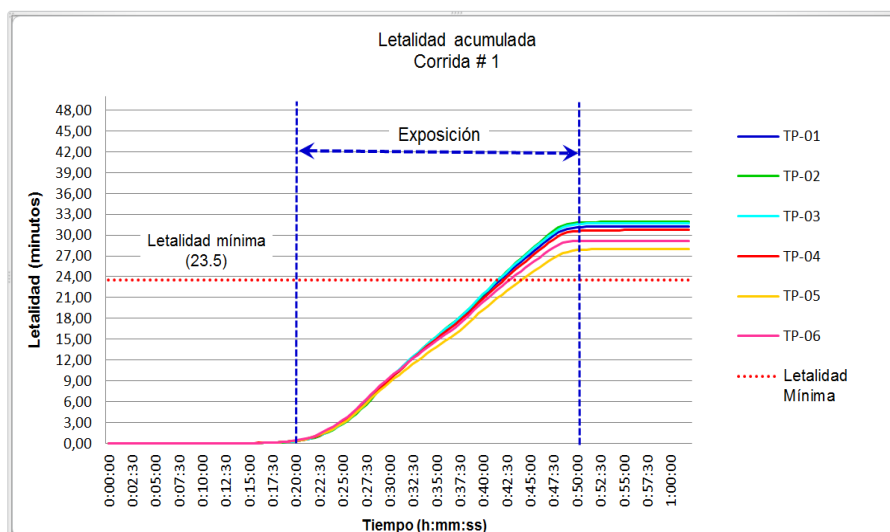
Fig. 4 Letalidad acumulada ( F_0 ) en la corrida 1 del Modo 3.
