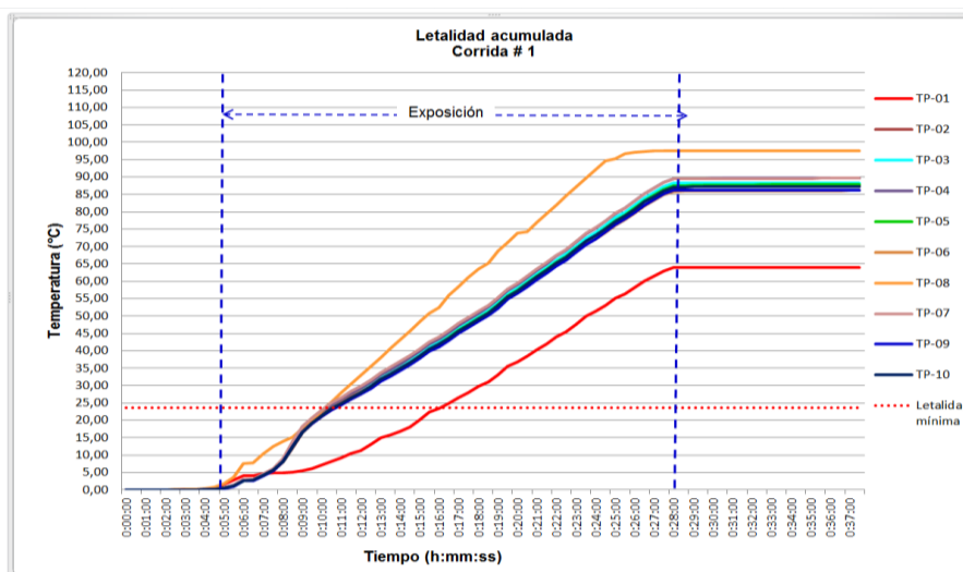
Fig. 2 Letalidad acumulada Modo 2.
