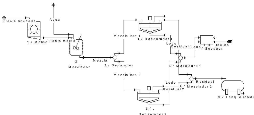
Fig. 4 Esquema tecnológico de la planta de producción de inulina a partir de la Tuna
