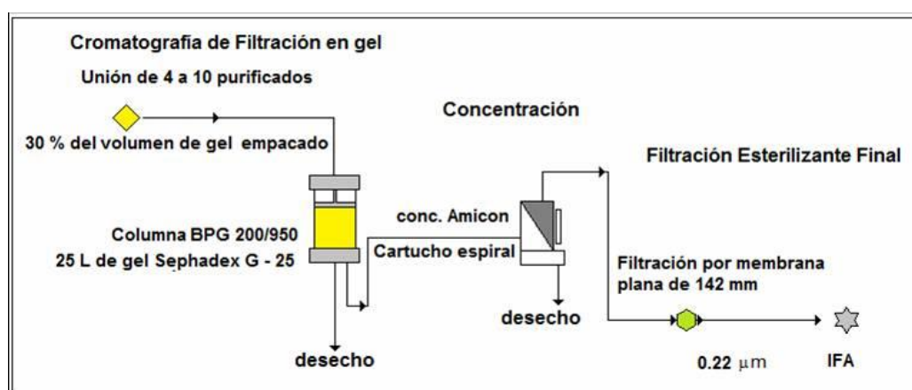
Fig. 5. Esquema de Flujo de la etapa de Conformación del IFA
