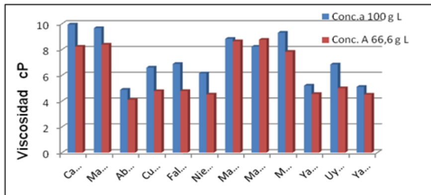
Fig. 1 Comportamiento de la viscosidad de las soluciones sin los balsos.
