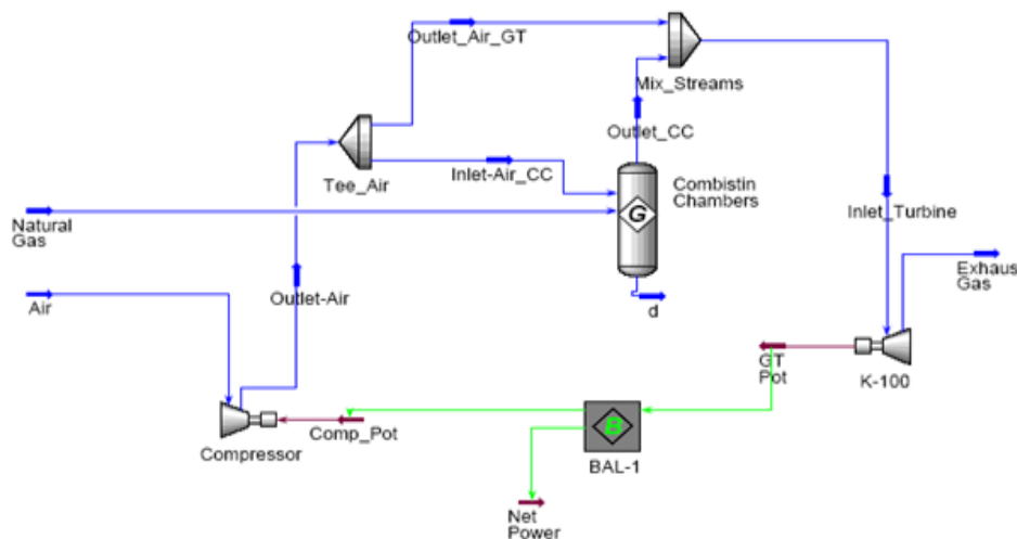
Fig. 3 Diagrama de flujo de información del ciclo de turbina de gas con regeneración en HYSYS.
