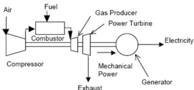
Fig. 1 Esquema representativo de un ciclo de turbina de gas simple.
