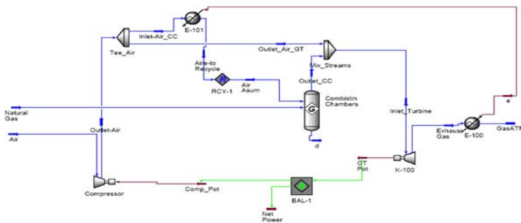
Fig. 2 Diagrama de flujo de información del ciclo de turbina de gas simple en HYSYS.
