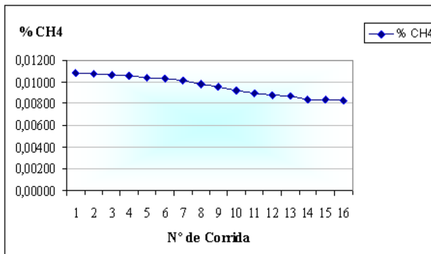
Fig. 3 Influencia de la variación en la calidad el LPG sobre el metano.
