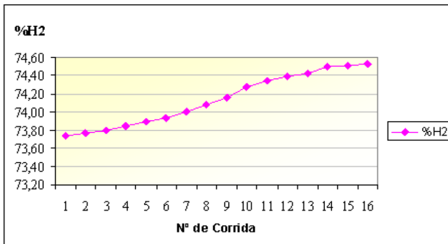
Fig. 2 Influencia de la variación en la calidad el LPG sobre el hidrógeno.
