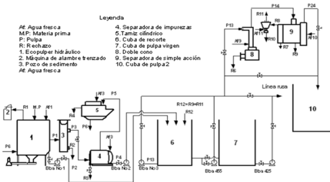
Fig. 2 Diagrama de flujo de la línea de preparación de pasta adquirida.
