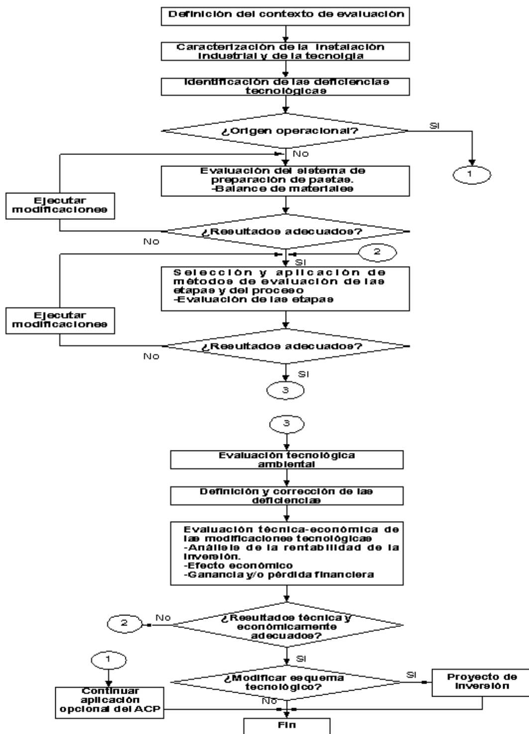
Fig. 1 Estrategia para la evaluación tecnológica del sistema de preparación de pastas.
