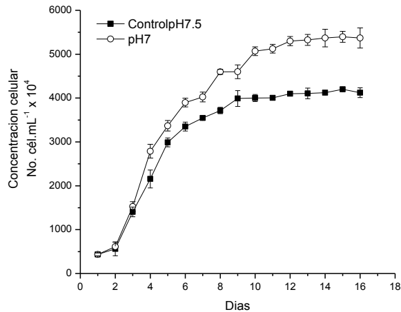
Fig. 6- Cinética de crecimiento en cultivos de 1L establecidos a pH 7 y 7,5 (Control) con la cepa local de Chlorella vulgaris
