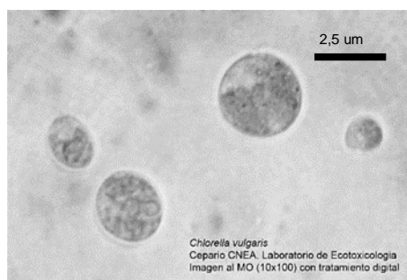
Fig. 1- Células de Chlorella vulgaris . Cepario del Laboratorio de Ecotoxicología del Centro Nacional de Electromagnetismo Aplicado (CNEA). Código: F010102-N
