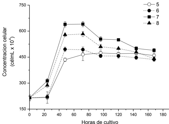
Fig. 2- Variación de la concentración celular con el pH en minicultivos no aireados de Chlorella vulgaris establecidos a 3000lx ( 58,59 \mu\text{E m}^{-2}\text{s}^{-1} )
