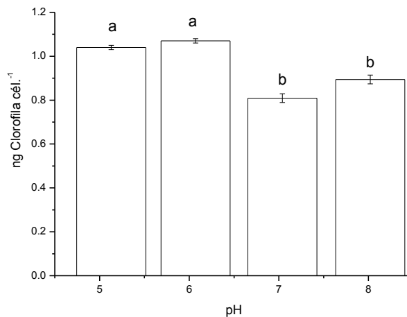
Fig. 5- Variación de la concentración de clorofila in vivo por célula a las 168h de cultivo. Letras diferentes corresponden a valores con diferencia estadísticamente significativas ( p=0,05 )
