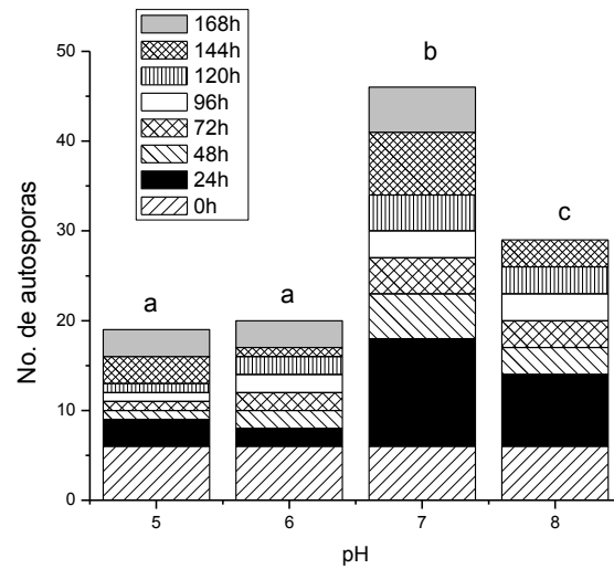
Fig. 4- Variación del número de autósporas con el pH (5 a 8u) durante las 168 h de cultivo (Serie 1: 0h, Serie 2: 24h, Serie 8: 168 h). Letras diferentes corresponden a valores con diferencia estadísticamente significativas ( p=0,05 )
