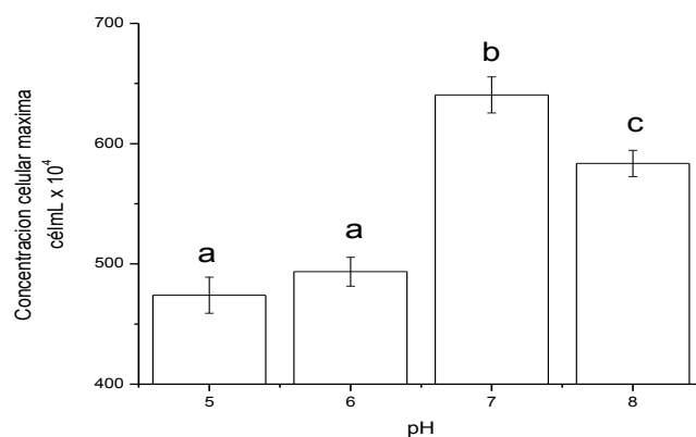
Fig. 3- Variación de la concentración celular máxima con el pH (5 a 8) en minicultivos no aireados de Chlorella vulgaris establecidos a 3000lx (58,59 \mu\text{E m}^{-2}\text{s}^{-1} ). Letras diferentes corresponden a valores con diferencia estadísticamente significativas ( p=0,05 )
