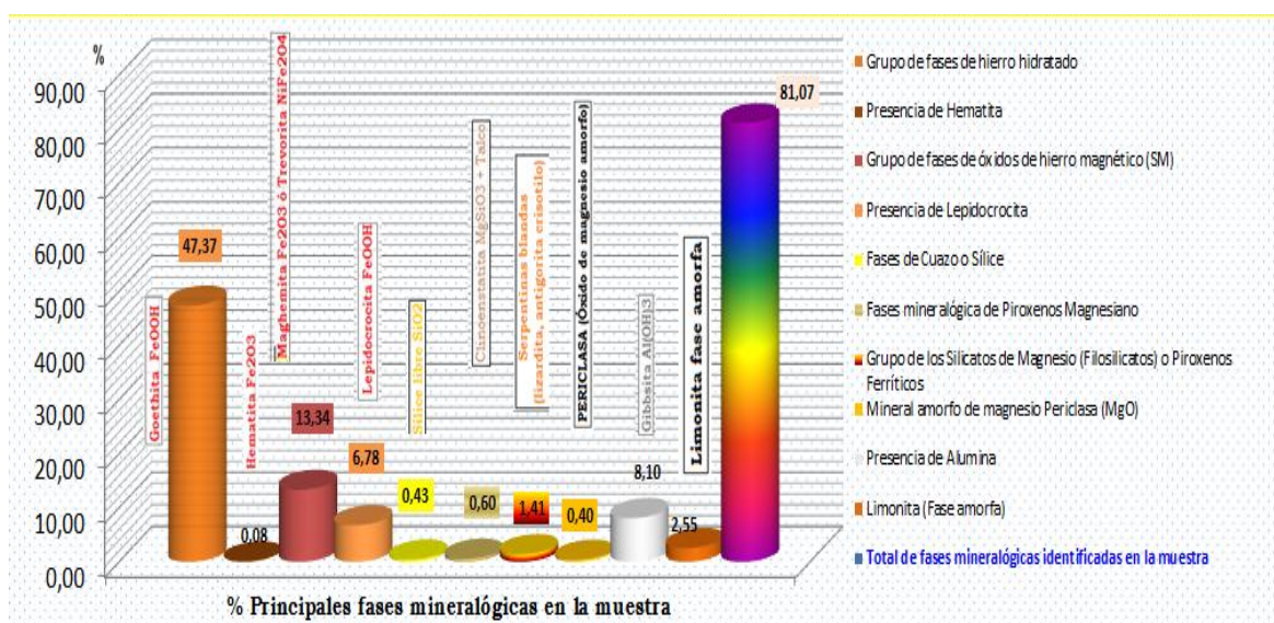
Fig.3- Mineralogía tecnológica de una mena comúnmente llamada limonítica o laterita natural
