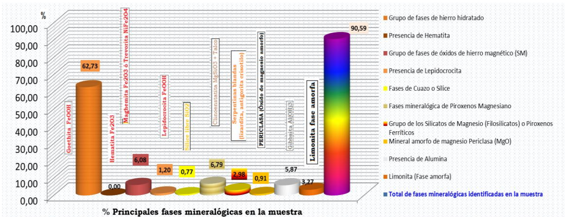
Fig. 4- Mineralogía tecnológica, de una mena con elevados contenidos de la fase de limonita y de la fase de silicatos de magnesio
