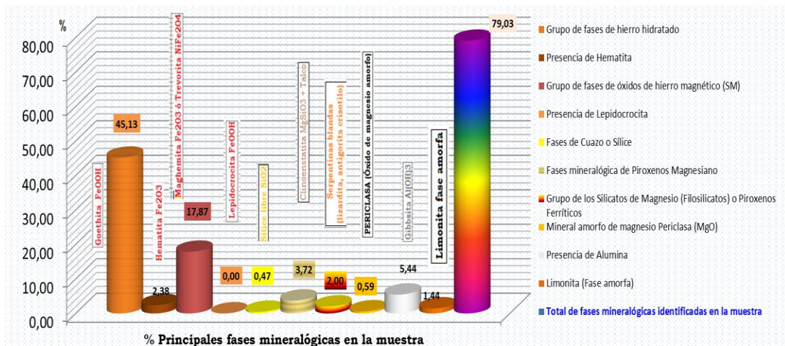
Fig. 5- Ejemplo de la mineralogía tecnológica de una mena de laterita de procesamiento industrial normal
