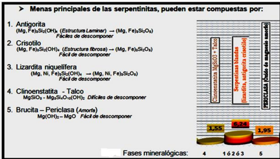
Fig. 2- Algunas fases mineralógicas de las menas serpentiniticas identificadas en forma de gráficos de barras
