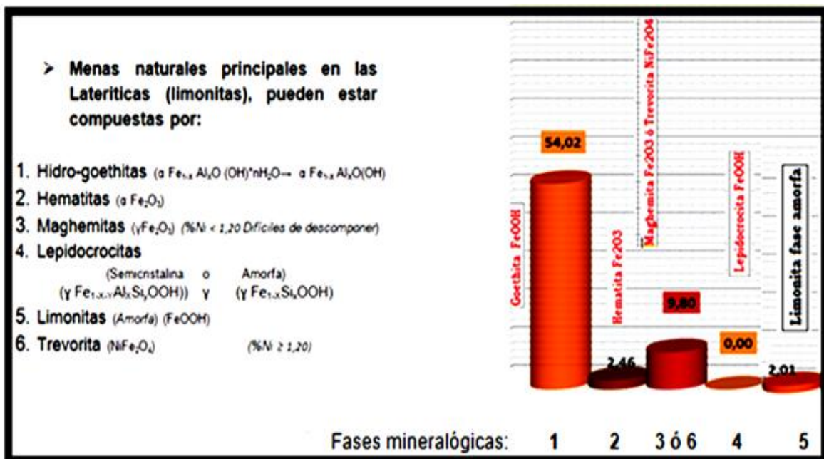
Fig. 1- Algunas fases mineralógicas de hierro identificadas en forma cuantitativa en un gráfico de barras de frecuencia
