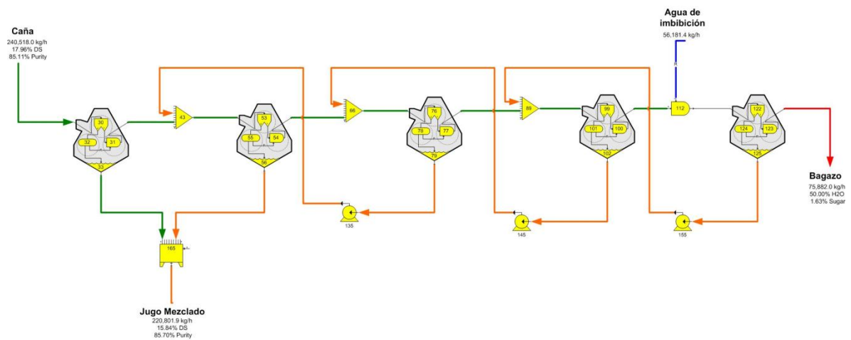
Fig. 5 - Esquema del área de Molinos
