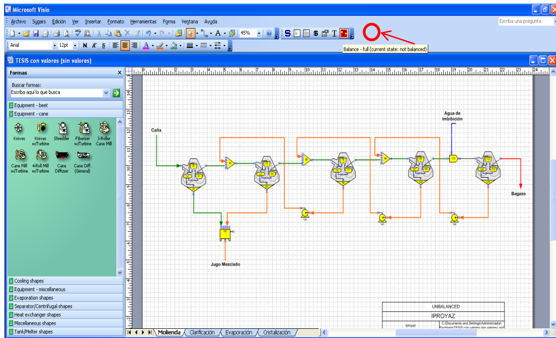
Fig. 3- Balance del área de molinos
