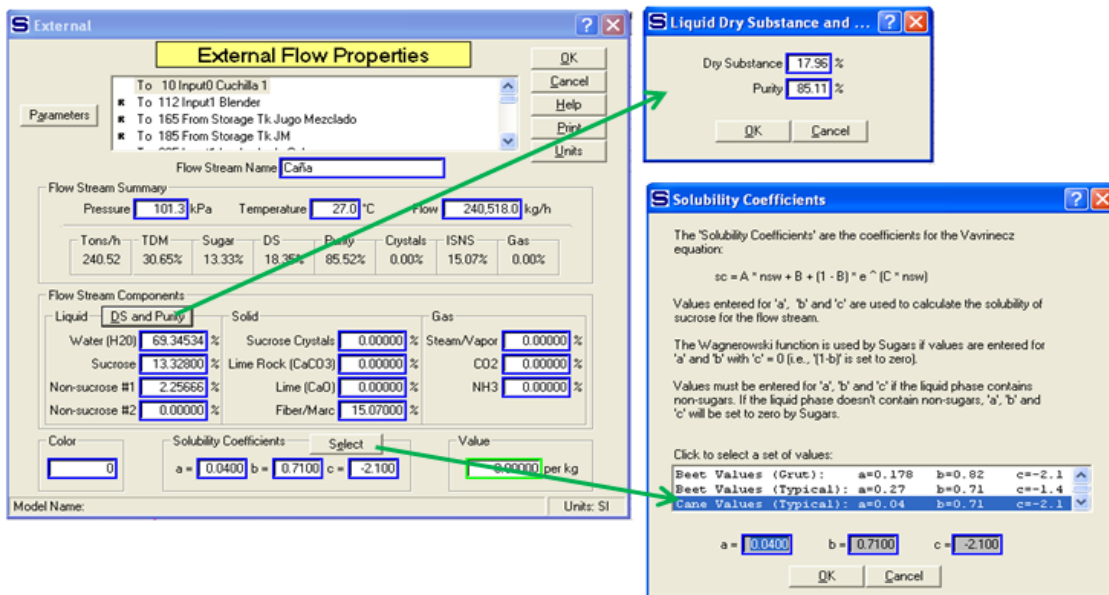
Fig. 1- Datos de la corriente de entrada
