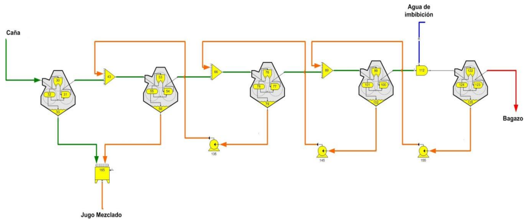
Fig. 2 -Esquema de equipos tecnológicos.
