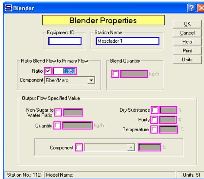
Fig. 4- Parámetro de operación del mezclador 1
