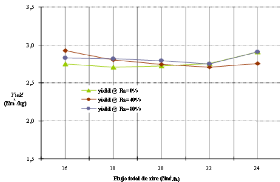
Fig. 1 Capacidad de producción de gas por unidad de biomasa alimentada (Yield) para R_a = 0, 40 y 80\% .
